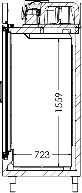
SECTION A-A
